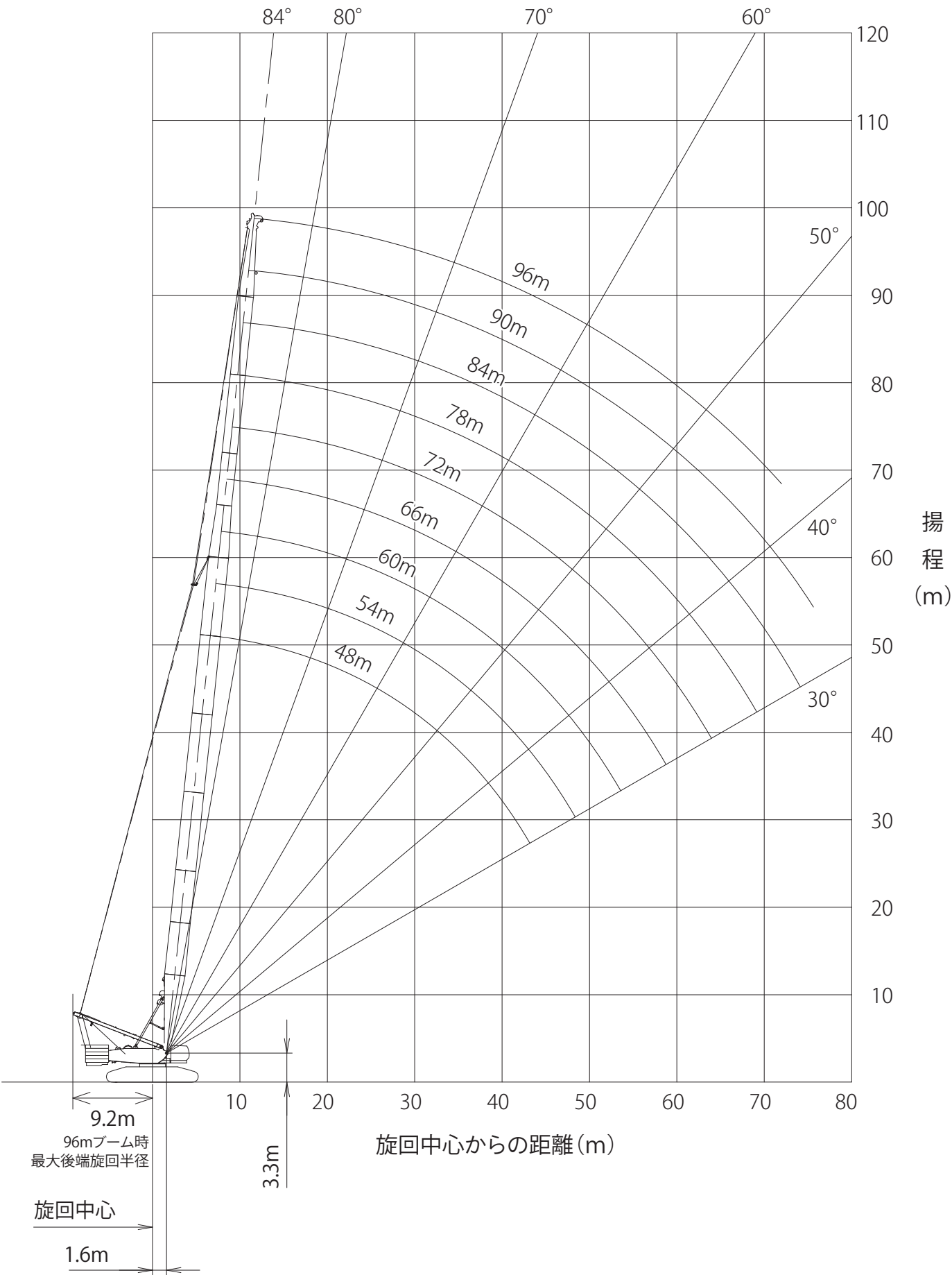
▶ ロングブーム作動範囲図
